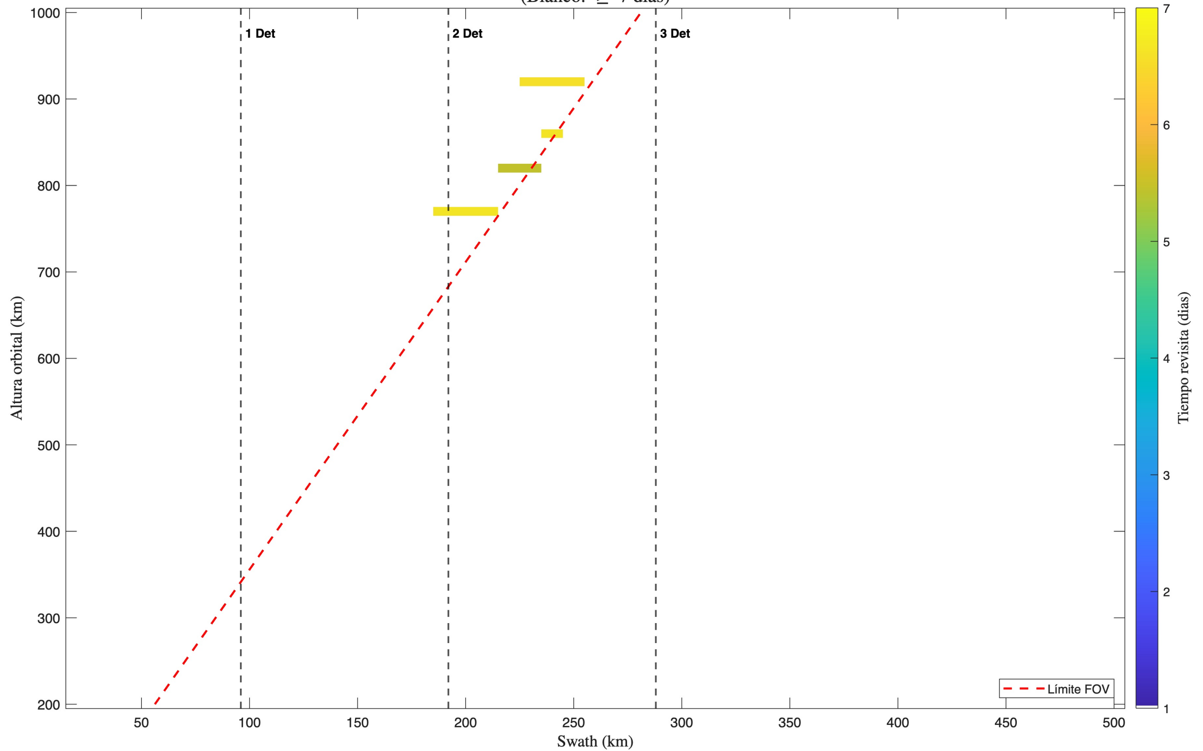
Tiempo Revisita - 2 Satelite(s); 2 Telescopio(s): TMA; Detector 1 (Blanco: \geq 7 dias)
